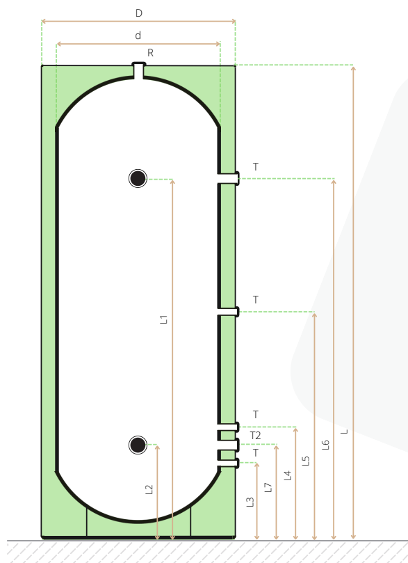
Rzut I - główny z izolacją
